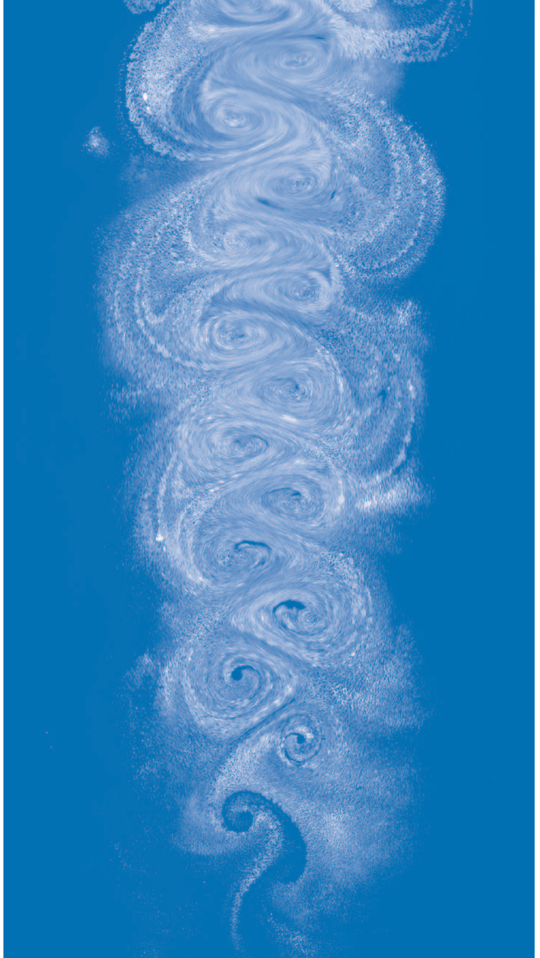
ABBILDUNG 3.2 Wirbelstraße in zäher Flüssigkeit (Aufsicht; siehe Versuch 3.1).
